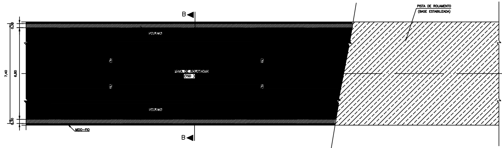
PAVIMENTAÇÃO – RUAS COM LARGURA DE 7,40m – RUA BURITI e RUA CEDRO PISTA SIMPLES COM SARJETA PLANTA ESC. 1:150
