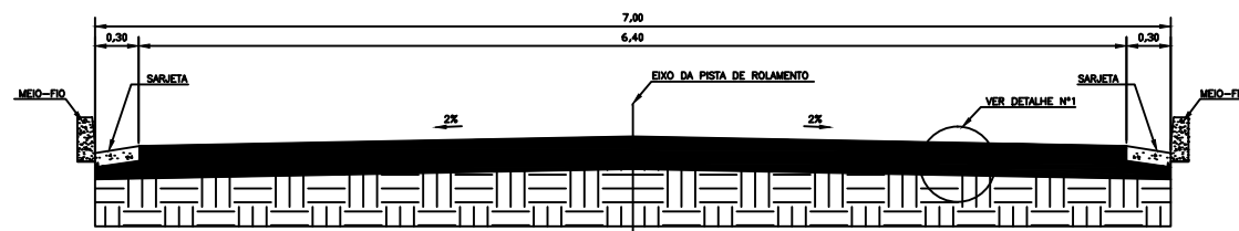
SEÇÃO TRANSVERSAL TIPO – BB ESC. 1:50
