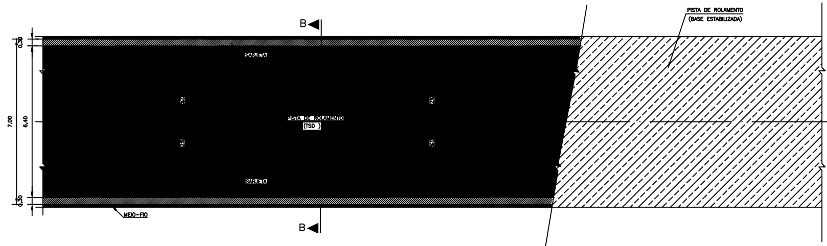
PAVIMENTAÇÃO – RUAS COM LARGURA DE 7,00 – RUA IPÊ (ENTRE BURITI e CEDRO) PISTA SIMPLES COM SARJETA PLANTA ESC. 1:150
